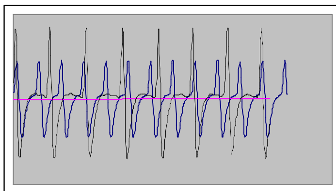
شکل ۱. تاثیر ۱ میکرو مولار E-4031 بر فعالیت خود به خودی یک دوره قلبی گره سینوسی-دهلیزی. ثبت های خارج سلولی پتانسیل عمل کوتاهتر مربوط به حالت کنترل و ثبت های خارج سلولی پتانسیل عمل بلندتر مربوط به مصرف E-4031 می باشد. واحد اندازه گیری در محور عمودی (بلندی پتانسیل عمل) هزارم ولت و در محور افقی (زمان) هزارم ثانیه است.
