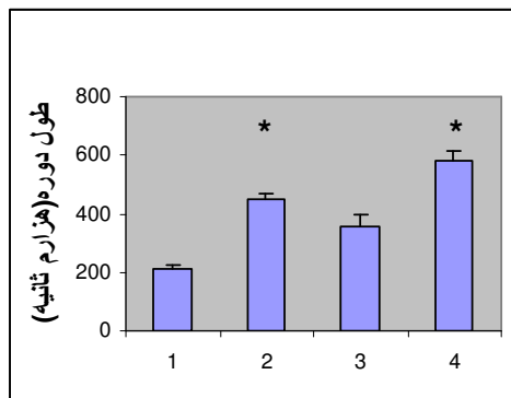
شکل ۲. مقایسه فعالیت خود به خودی دوره گره سینوسی-دهلیزی و دهلیزی-بطنی در حالت کنترل و مصرف ۱ میکرو مولار E-4031. ستون ۱ و ۲ به ترتیب مربوط به حالت کنترل گره سینوسی-دهلیزی و دهلیزی-بطنی، ستون ۳ و ۴ به ترتیب مربوط به مصرف دارو در گره سینوسی-دهلیزی و دهلیزی-بطنی است. * = تفاوت معنی دار ( p < 0.05 ) با گره سینوسی-دهلیزی.
